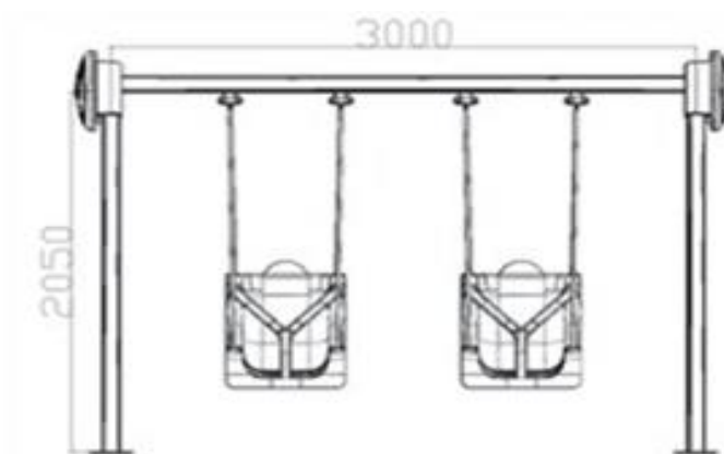
Фигура 3.2 Размер 2
