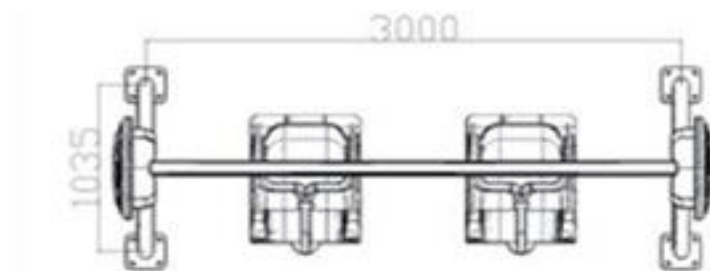
Фигура 3.1 Размер 1
