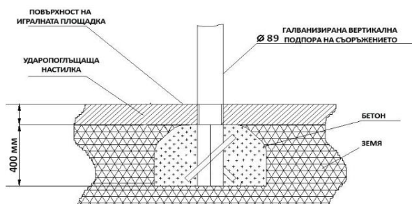
Фигура 5.2 Фундаментна скица на подпорите
