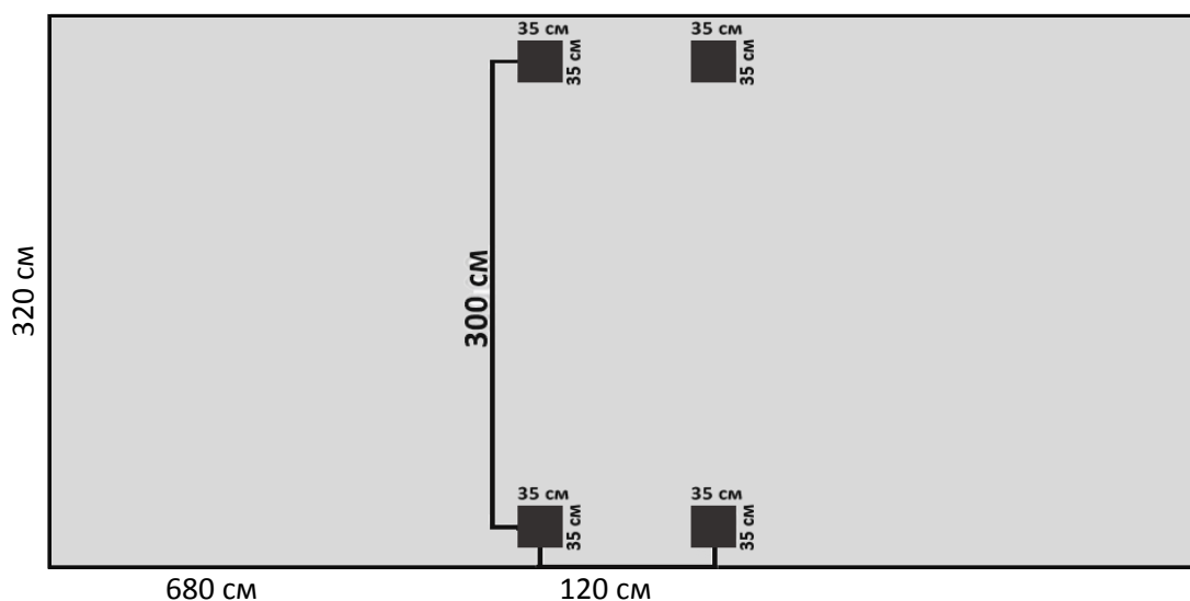
Фигура 5.1 Фундаментна скица
